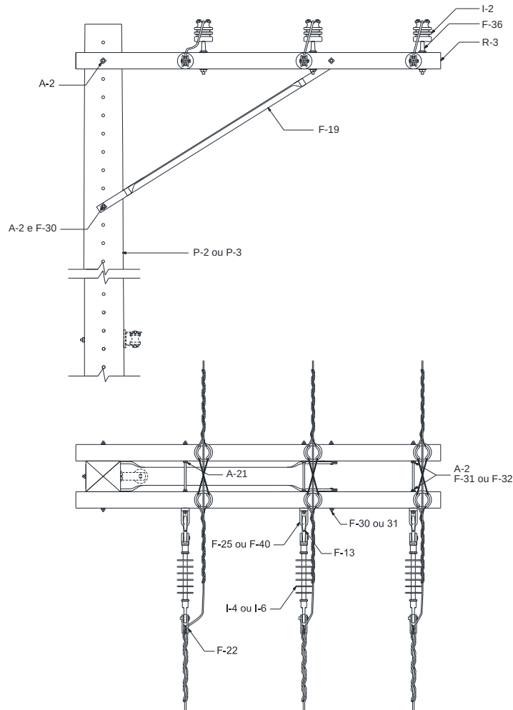
Figura 64 – Estrutura B3-2 – Poste de seção DT ou de madeira
