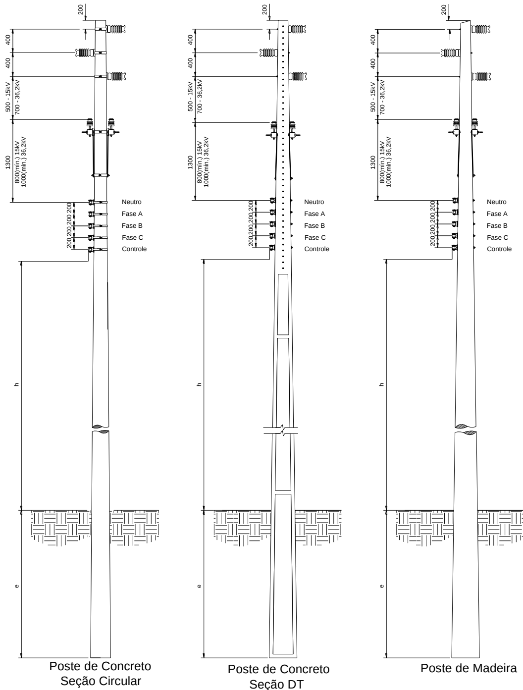
Figura 14 – Afastamentos mínimos – Estruturas pilar trifásicas tangentes com derivação
